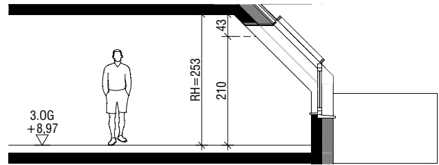
SCHNITT A
