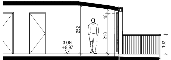
SCHNITT B
