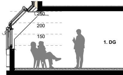
Schnitt
