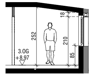
SCHNITT B
