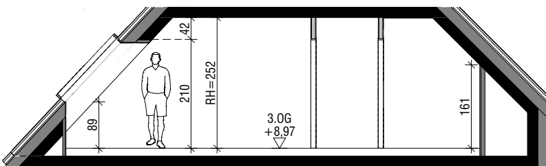
SCHNITT A
