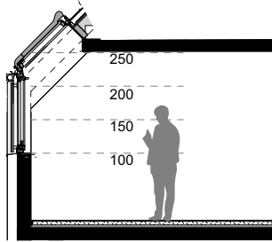
Schnitt
